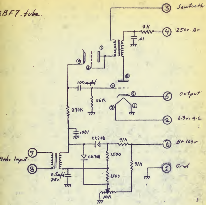
FIG. 4 - PRC MODULATOR
