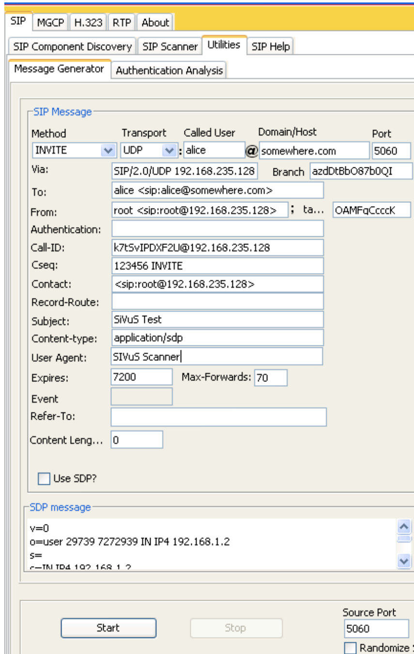
Figure 15. SiVus message generation screen
