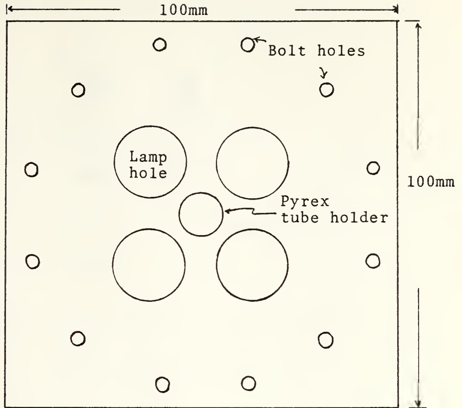
Fig. 12. End plate: Scale 1:1
