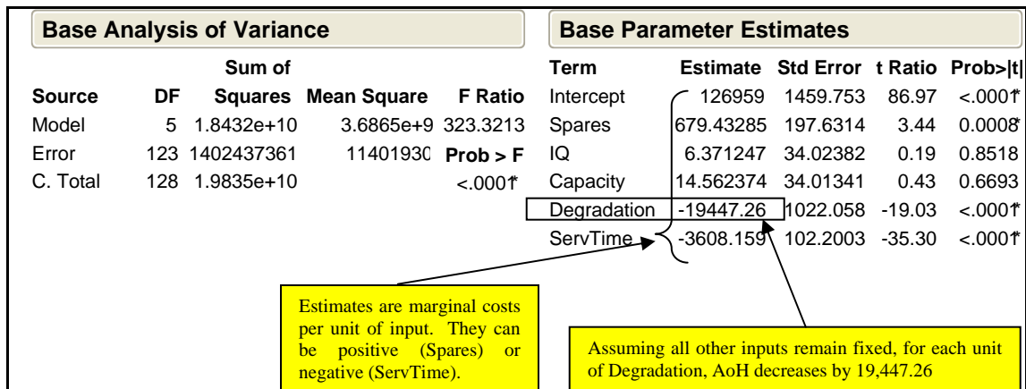
Figure 16. Baseline main parameter ANOVA and estimates
